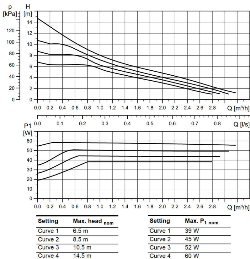
Charakterystyka Q(H)
